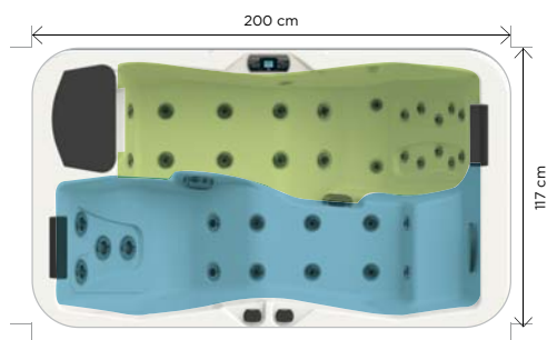
Höhe 78 cm / Fassungsvermögen: 450 l
