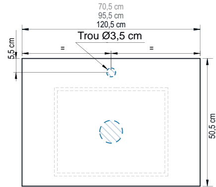
Trous pour l'évacuation du lavabo et le robinet
